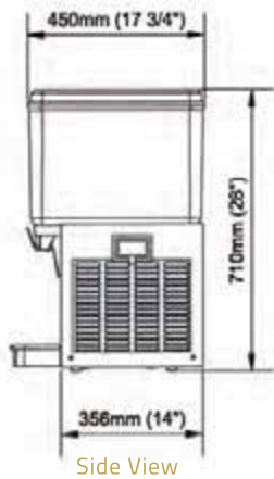
JD 118 MIX
